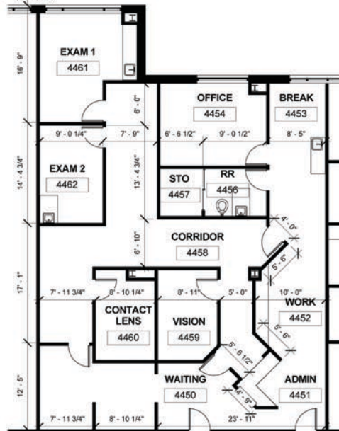
② STE 445 1/8" = 1'-0"
